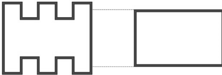
Abbildung 3.4 Darstellung eines stark gegliederten Grundrisses (links) und eines optimierten Grundrisses (rechts)
