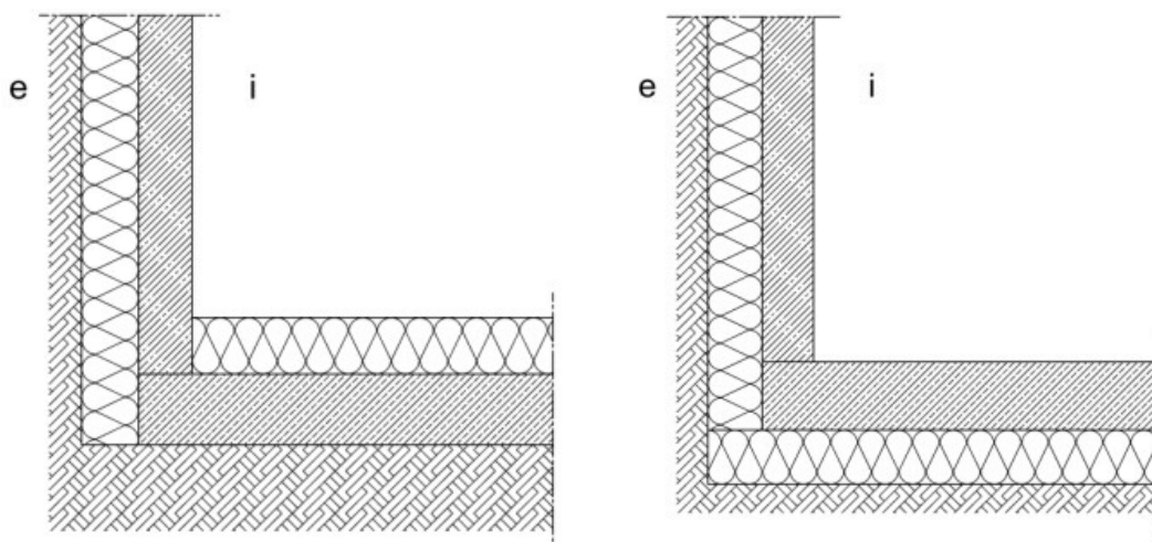
Abbildung 3.7 Darstellung einer „Dämm-lücke“ (links) und des optimierten Anschlusses (rechts)
