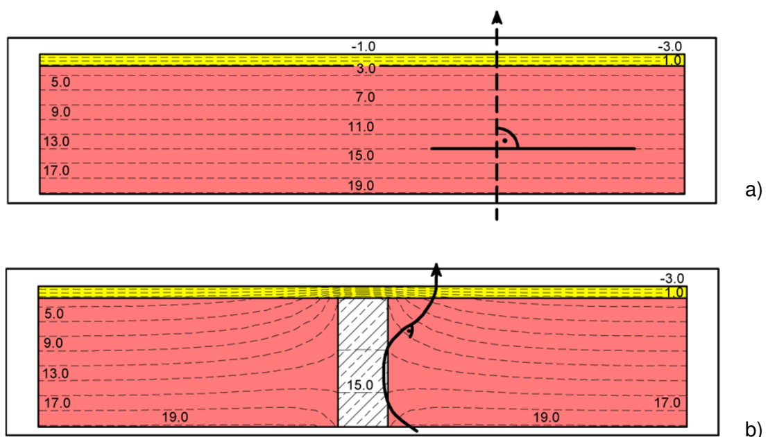
Abbildung 3.2 Verlauf von Isothermen und Wärmestrom a) „ungestörter“ und b) „gestörter“ Bereich
