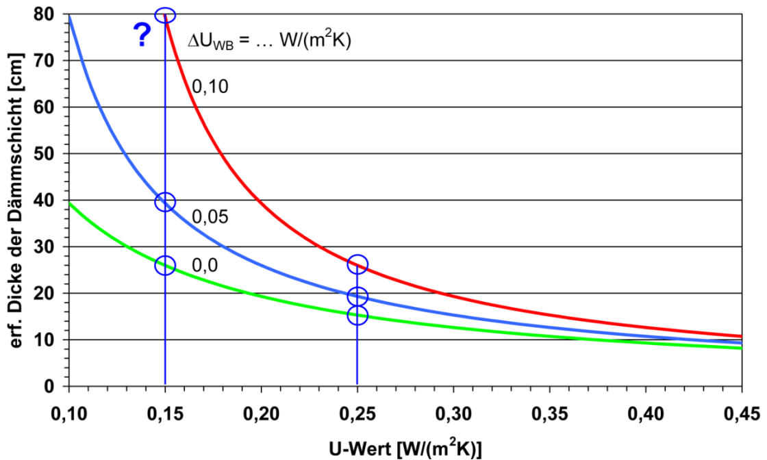
Abbildung 3.3 Beeinflussung der erforderlichen Dämmschichtdicken durch den Wärmebrückenzuschlag \Delta U_{WB}
