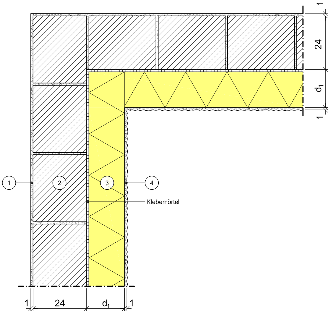
Horizontalschnitt
