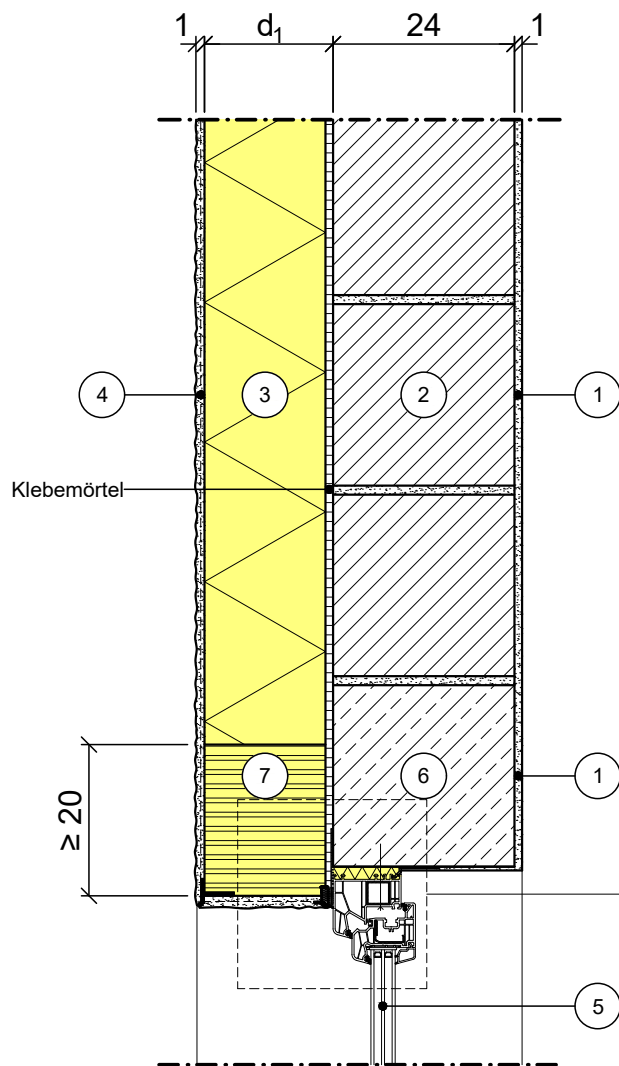
Vertikalschnitt
